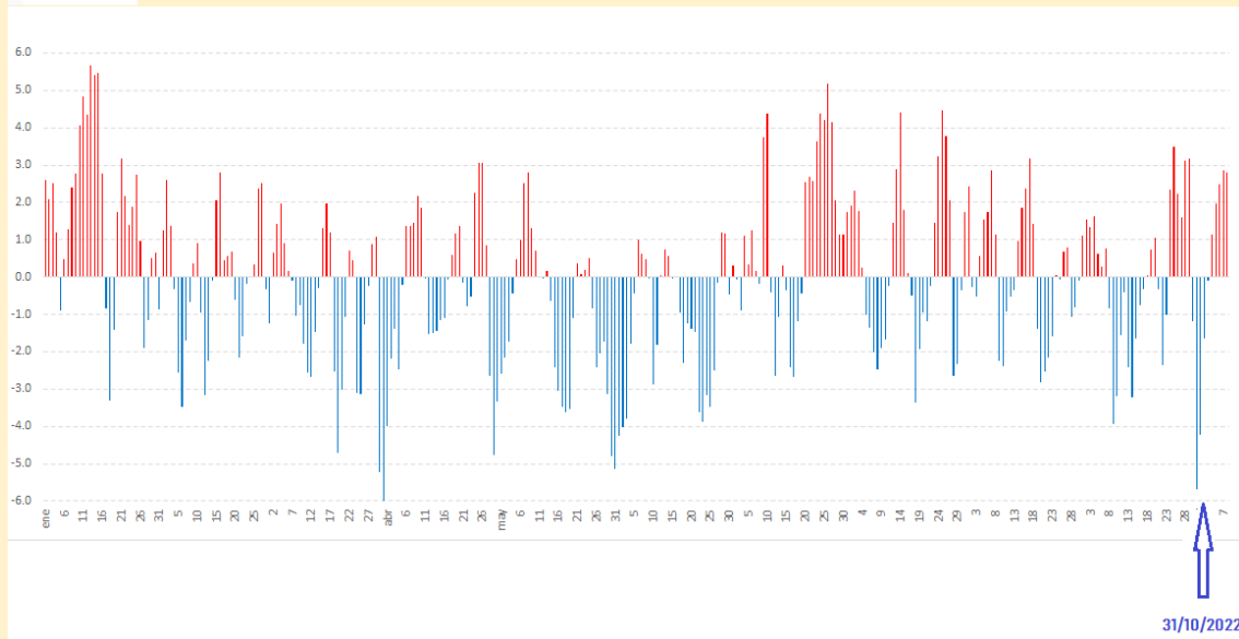
Anomalías de temperatura diaria (Arg.) 2022. Fuente: SMN
